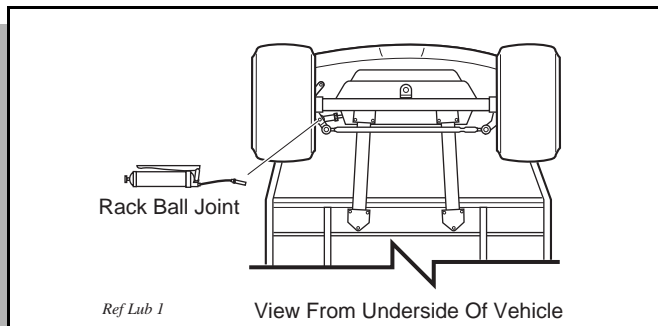
Fig. 37 Lubrication Points
