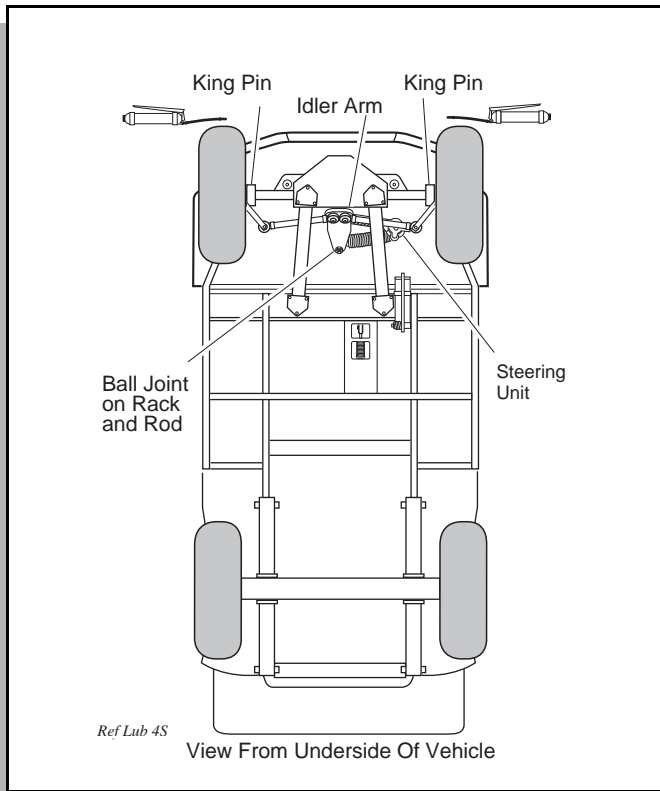
Fig. 32 Lubrication Points
